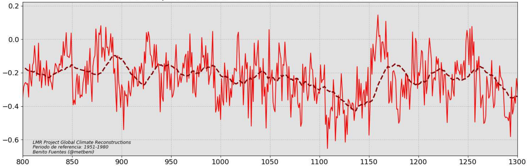
anomalía de temperatura ( ° C) en las islas británicas durante el Periodo Cálido Medieval
