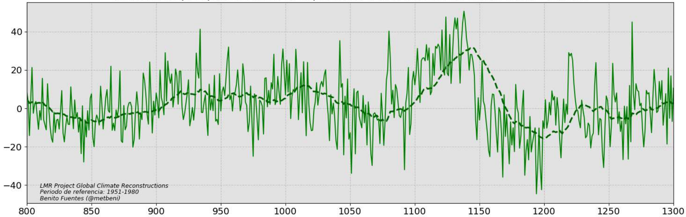
anomalía de precipitación (mm) en la península ibérica durante el Periodo Cálido Medieval
