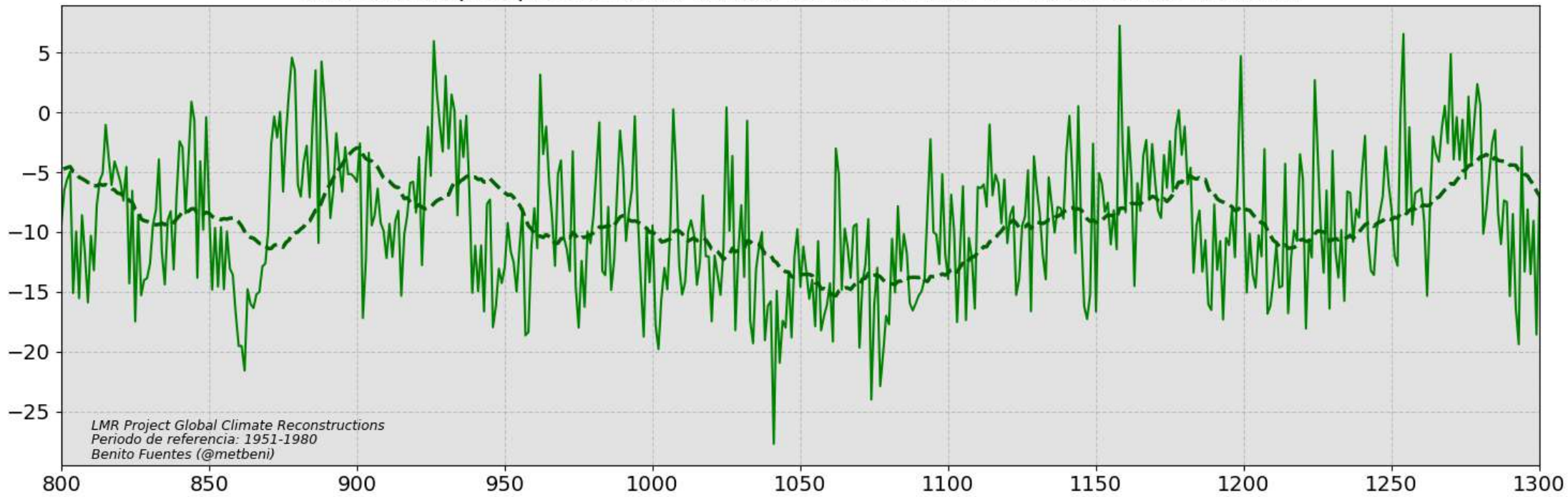
anomalía de precipitación (mm) en Asia Central durante el Periodo Cálido Medieval
