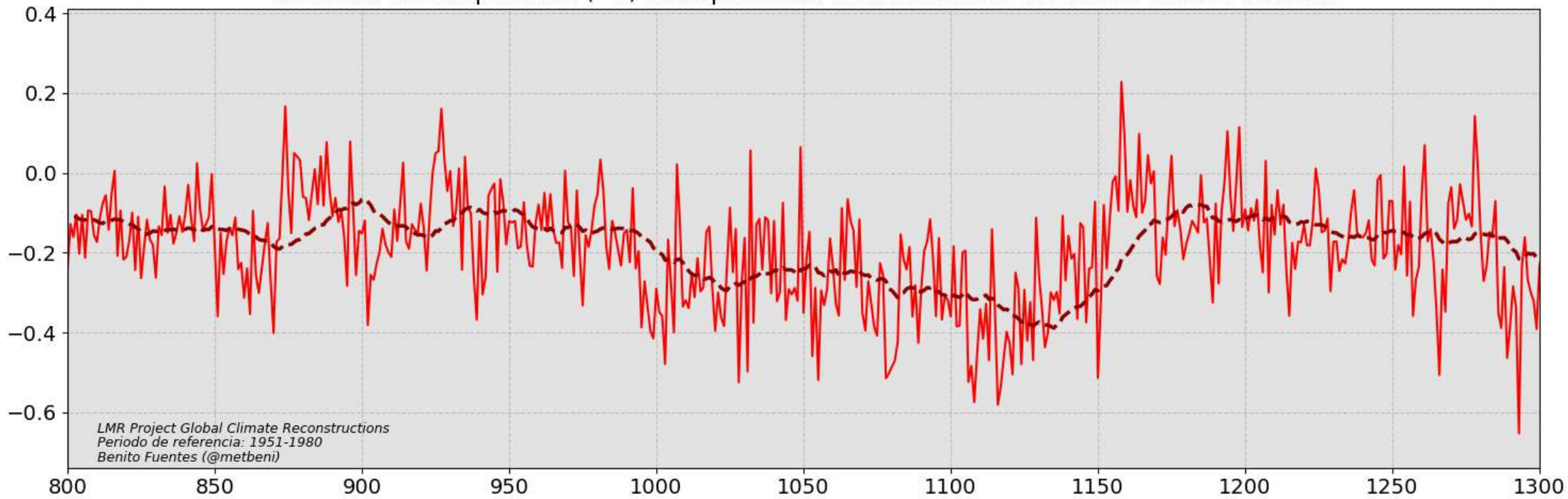
anomalía de temperatura ( ° C) en la península ibérica durante el Periodo Cálido Medieval
