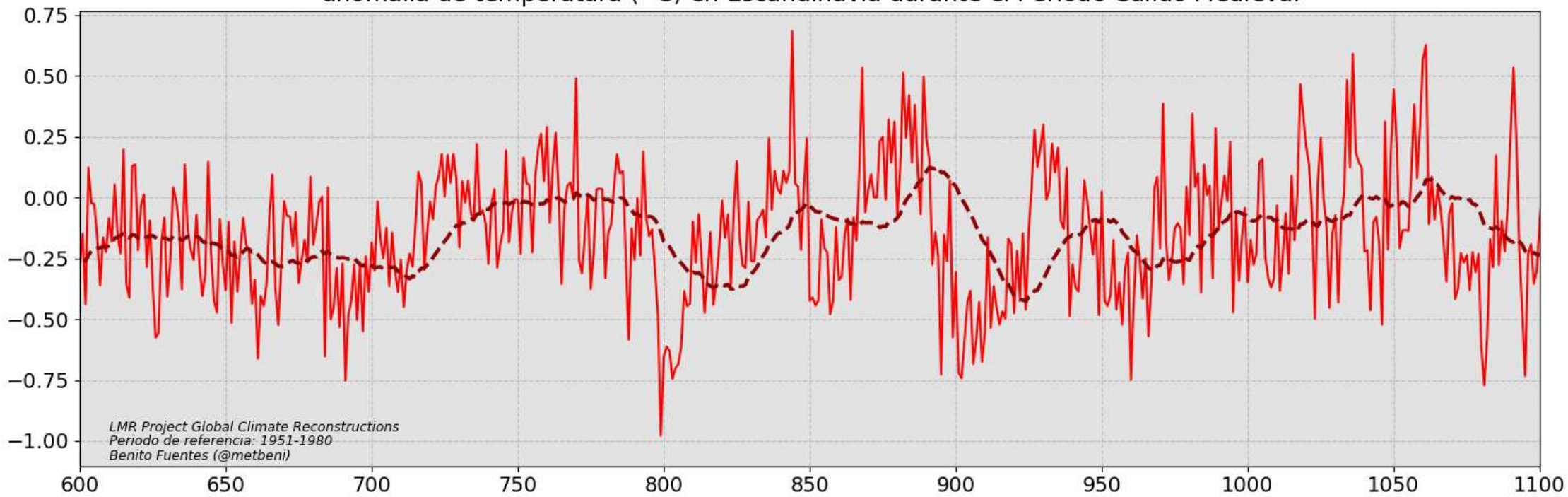
anomalía de temperatura ( °C) en Escandinavia durante el Periodo Cálido Medieval
