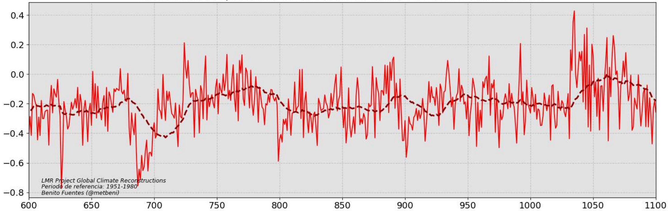
anomalía de temperatura ( ° C) en Terranova durante el Periodo Cálido Medieval
