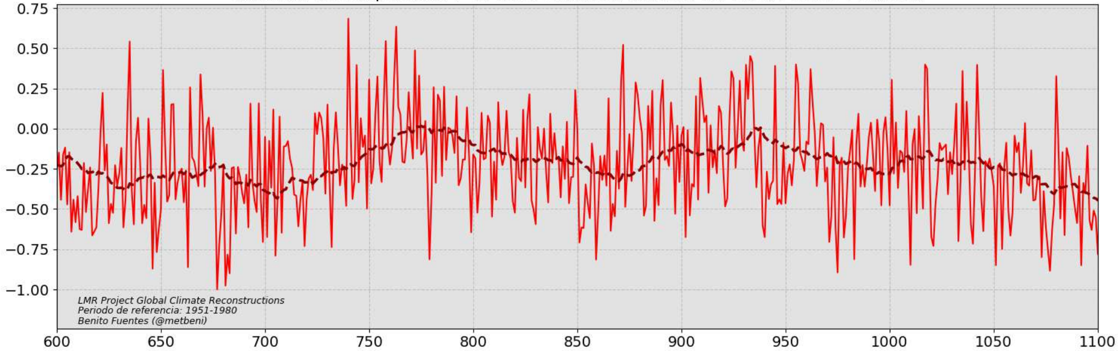
anomalía de temperatura ( °C) en Groenlandia durante el Periodo Cálido Medieval
