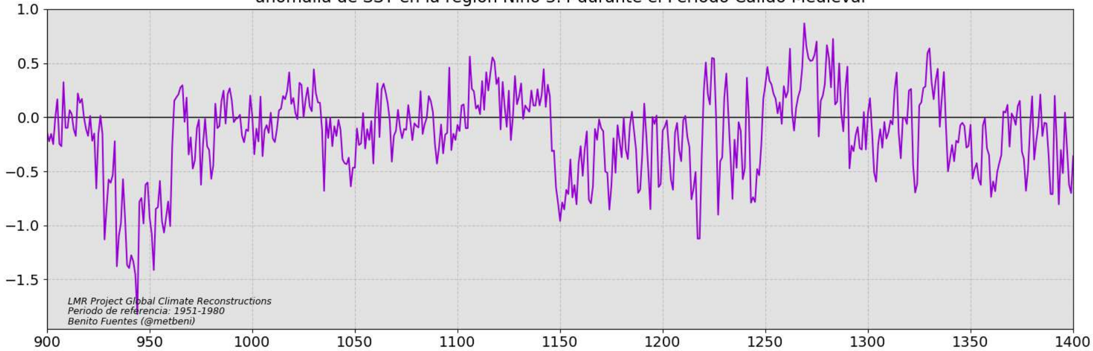
anomalía de SST en la región Niño 3.4 durante el Periodo Cálido Medieval
