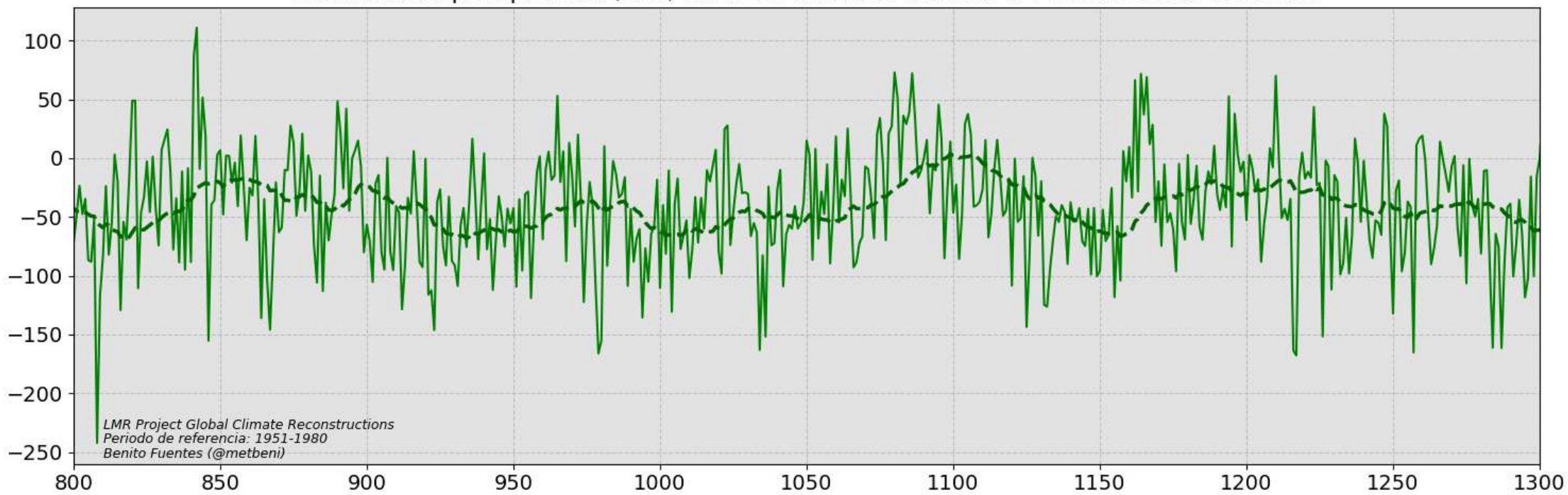
anomalía de precipitación (mm) en el SW de EEUU durante el Periodo Cálido Medieval
