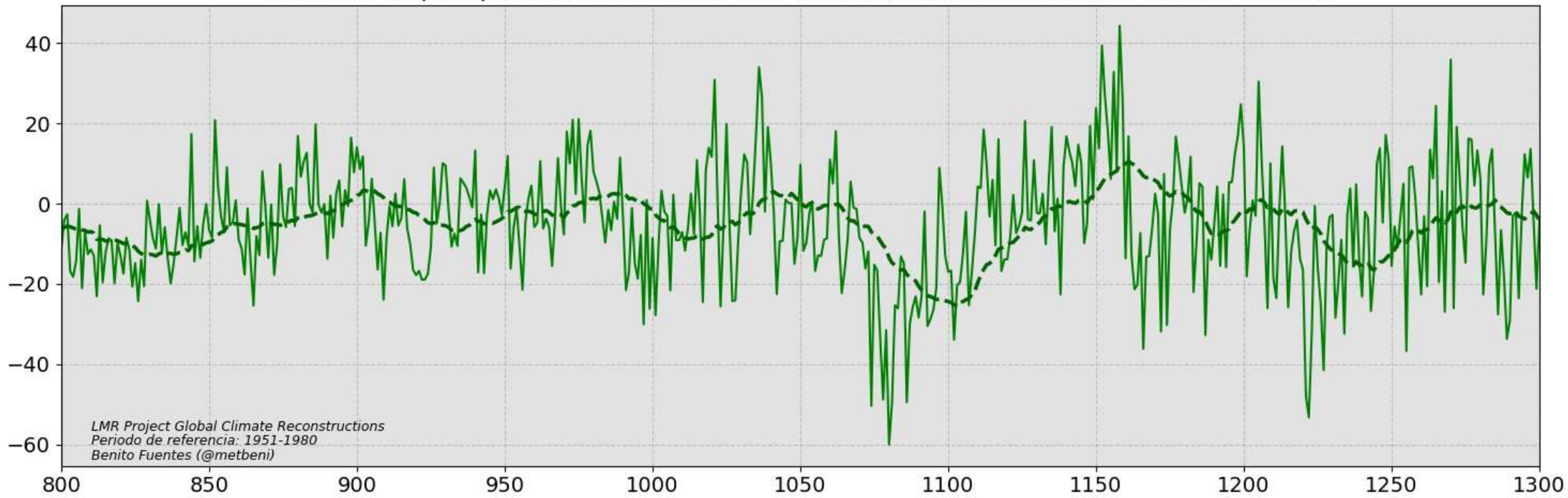
anomalía de precipitación (mm) en las islas británicas durante el Periodo Cálido Medieval
