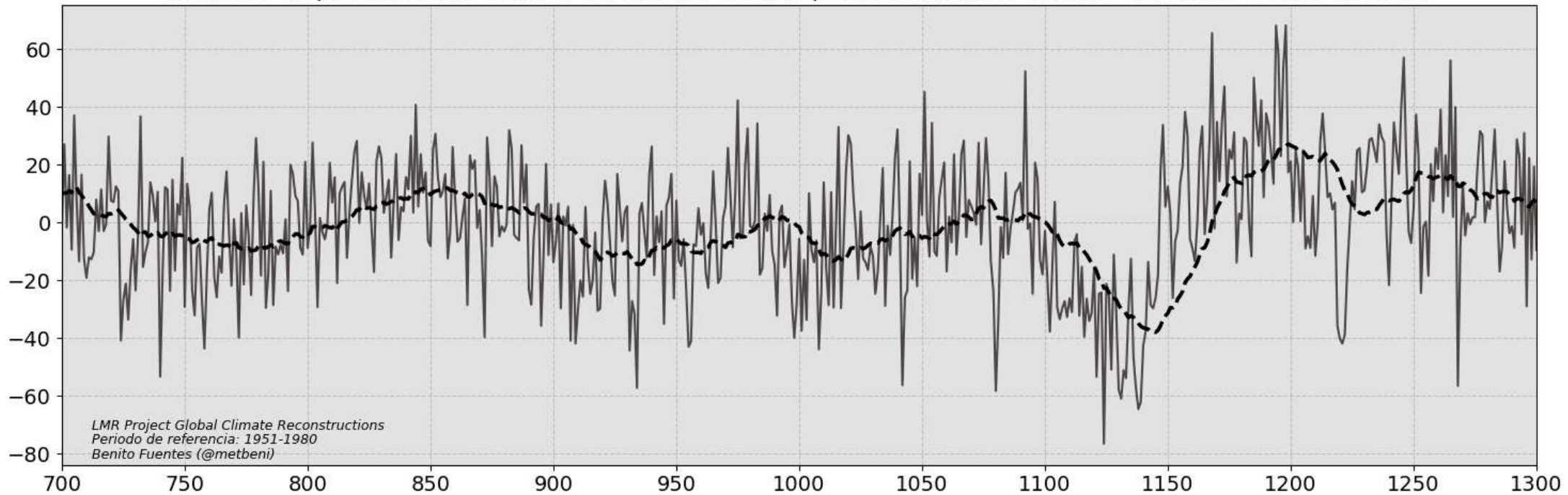
anomalía de presión sobre el nivel del mar (hPa) en la península ibérica durante el Periodo Cálido Medieval
